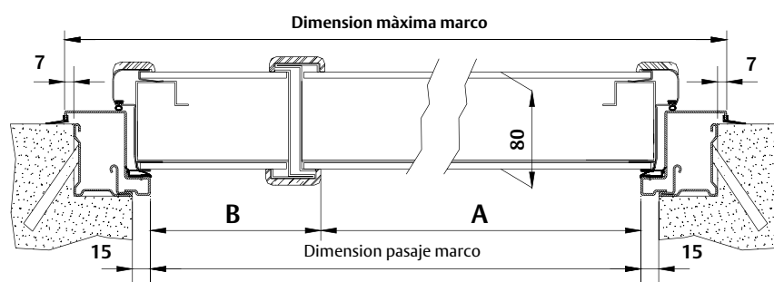
SECCIÓN HORIZONTAL
